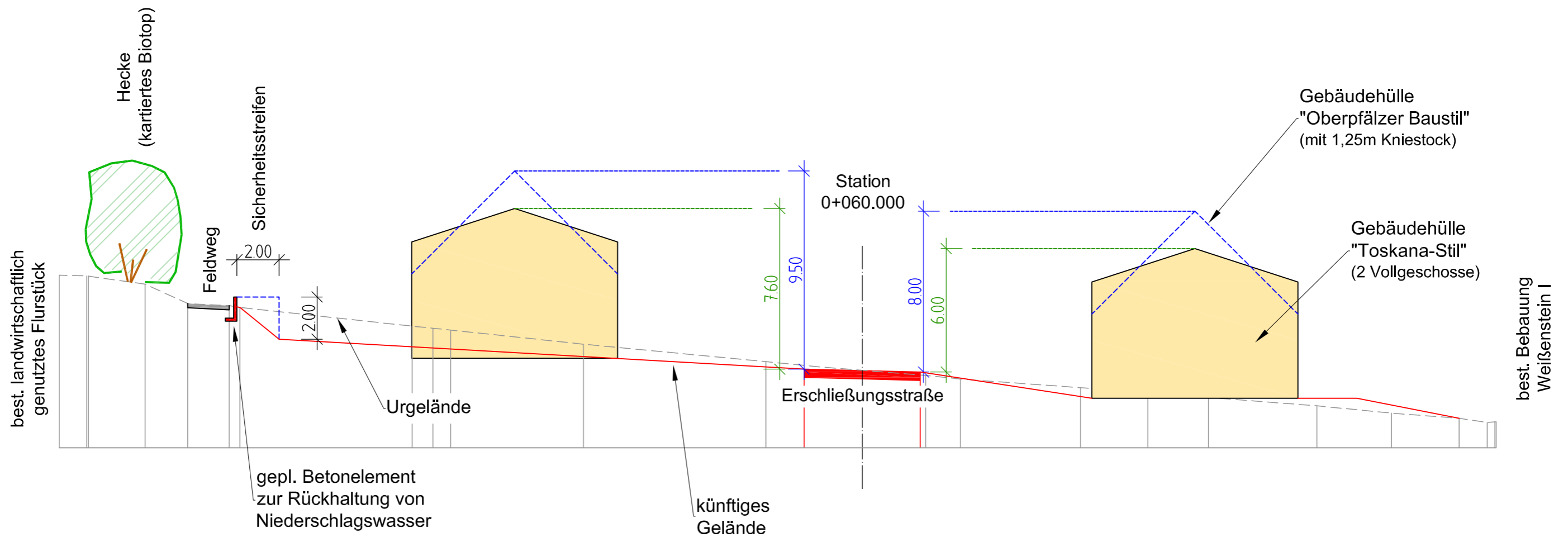
Systemschnitt bei Station 0+060 (mit Blick Richtung Osten - Maßstab 1 : 200)
